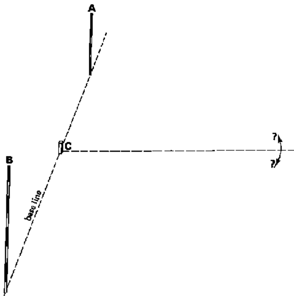
شکل ۲۱ الف. د قائمه زاویې جوړول ، لومړۍ مرحله Step 1 Fig. 21a Setting out a right angle,
