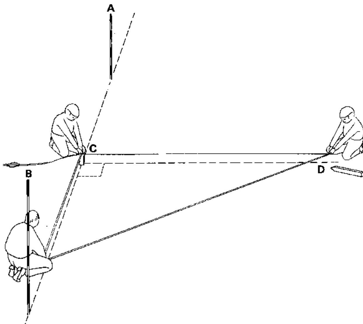
۲۱ (ب) شکل د قایمه زاویې ترسیم، دوهم مرحله Fig. 21b Setting out a right angle, Step 2
