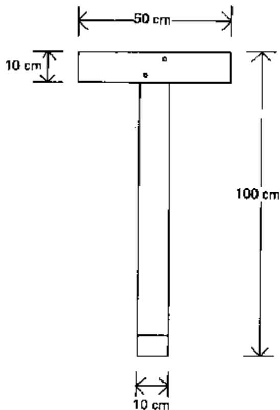
Fig. 34 A boning rod
