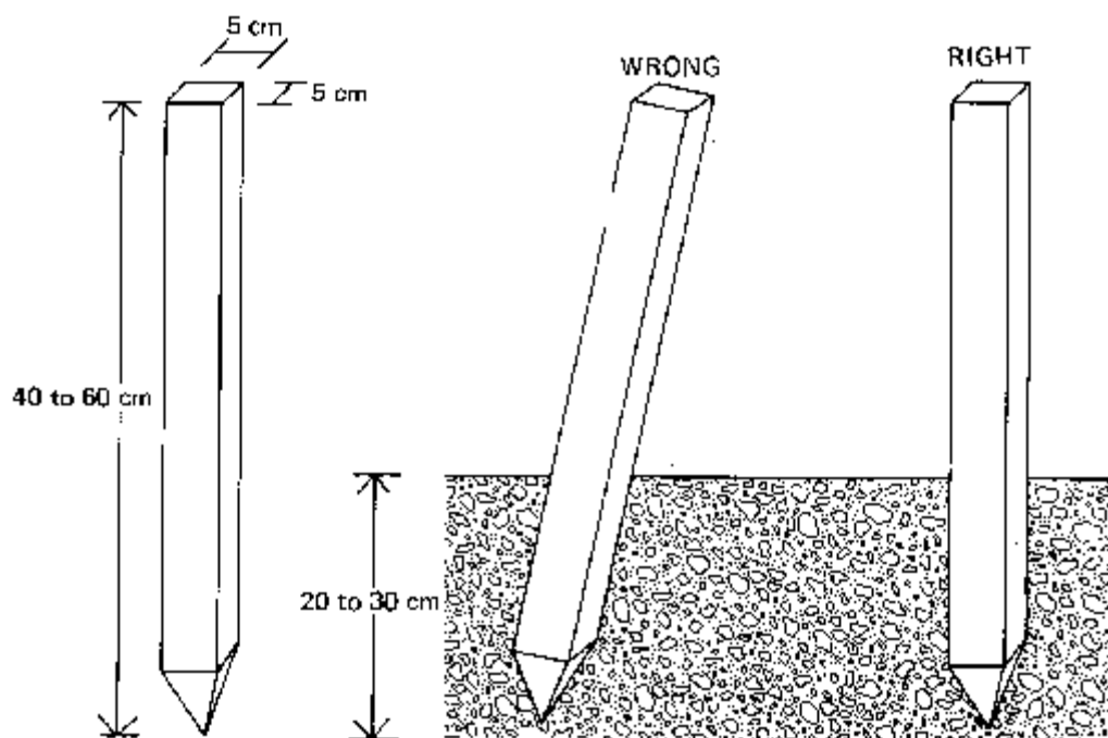
۸ شکل مړوی یا چوبی میخ Fig. 8 Pegs
