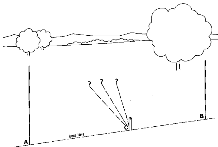
Fig. 27 Setting out a right angle ترسیمول د قائمه زاویي شکل ۲۷
